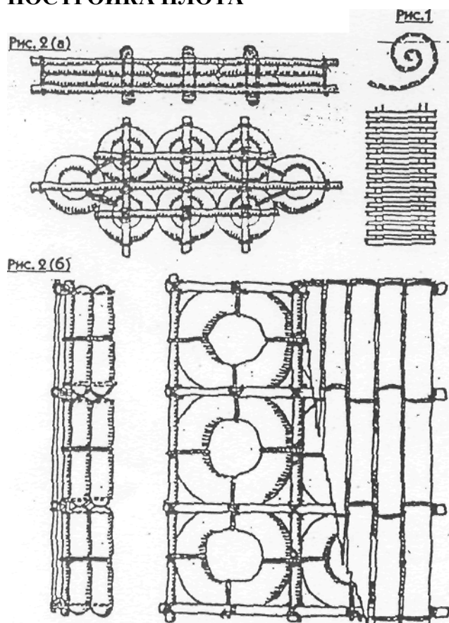
Постройка плота из автомобильных камер: Рис.1 Скручивающийся пол из реек. Рис.2а и рис. 2б Плоты разных типов - вид сверху и сбоку
