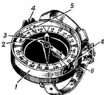
Рис. 10. Компас Адрианова:
